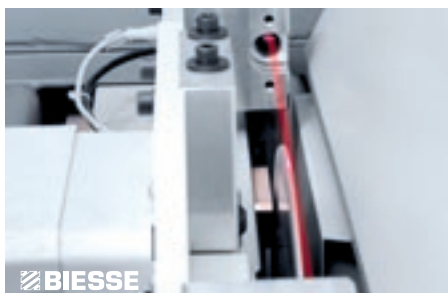
Dispositivo allineamento automatico dell'incisore delle sezionatrici Selco.
